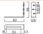
品名 タオレーズL型-1ヶ入 -2ヶ入 仕上:ユニクロ 材質:SPCC
