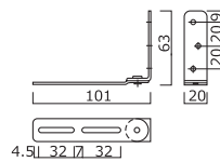
品名 タオレーズミニ-1ヶ入 -2ヶ入 仕上:クロメート 材質:SPCC
