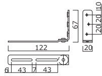
品名 タオレーズ-1ヶ入 -2ヶ入 仕上:黒 材質:SPCC
