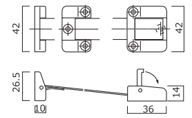
品名 タオレーズ BL-700 -2ヶ入 仕上:黒 材質:樹脂/ナイロン (本体/ベルト)
